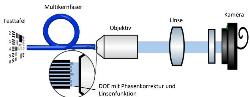
Schematischer Aufbau mit DOE
